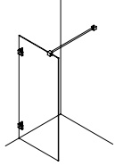
Typ 500 mit Wandwinkeln System Malta
